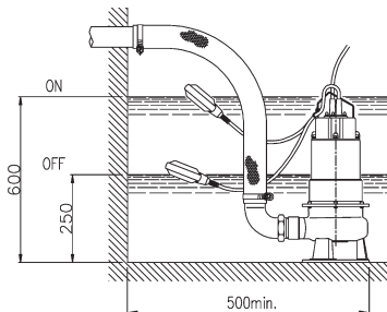
FIG. 7 • DW FZ VERSION
