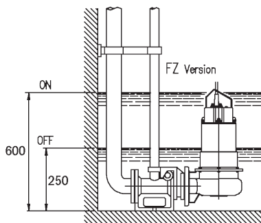
FIG. 7 • DW FZ VERSION
